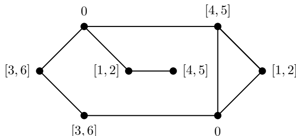
Fig. 2: A “ C_6 -amenable” graph G
