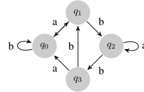
Fig. 1: A counterexample to Lemma 1
